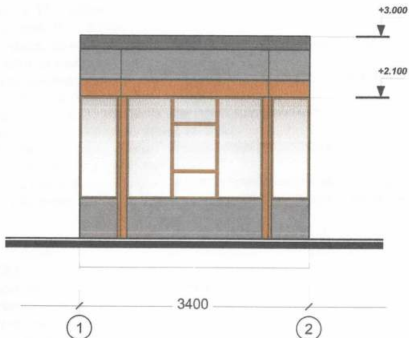
Бічний фасад
