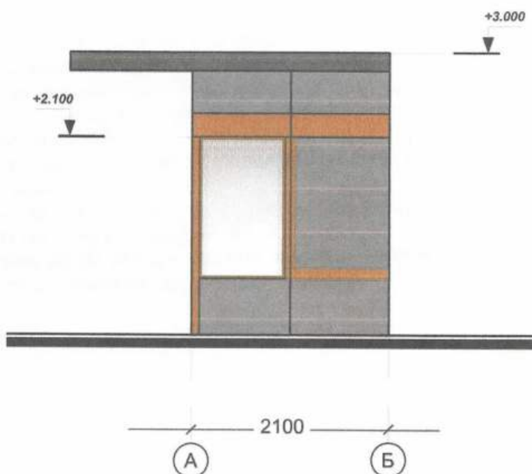
Бічний фасад
