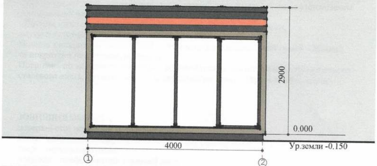
Боковий фасад
