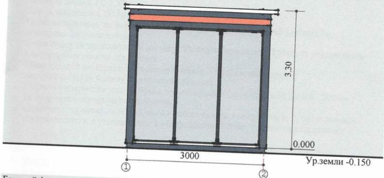
Боковий фасад
