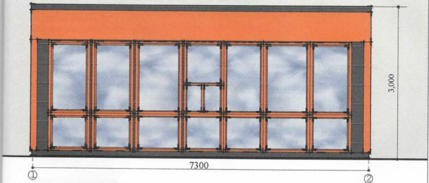
Боковий фасад
