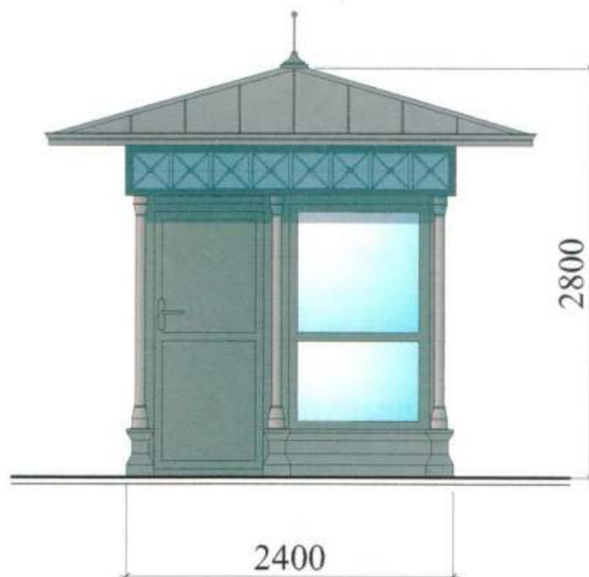
Бічний фасад ТС М 1:50
