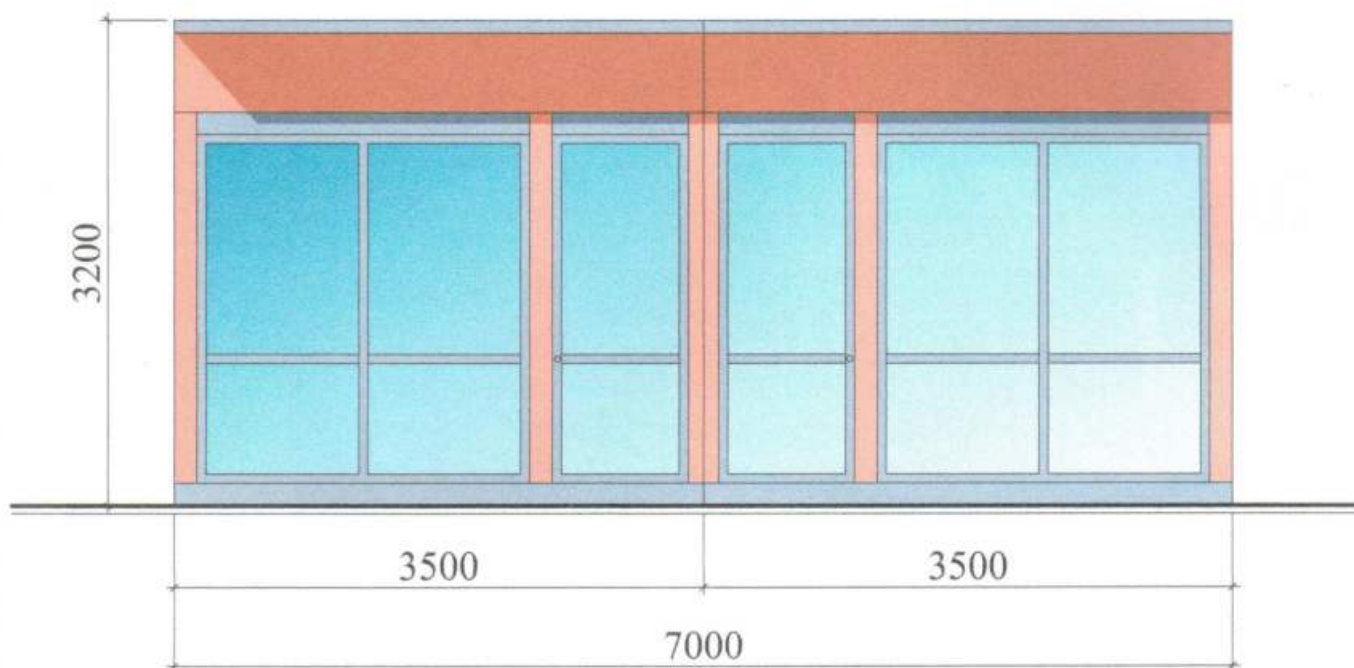
Головний фасад групи ТС М 1:50
