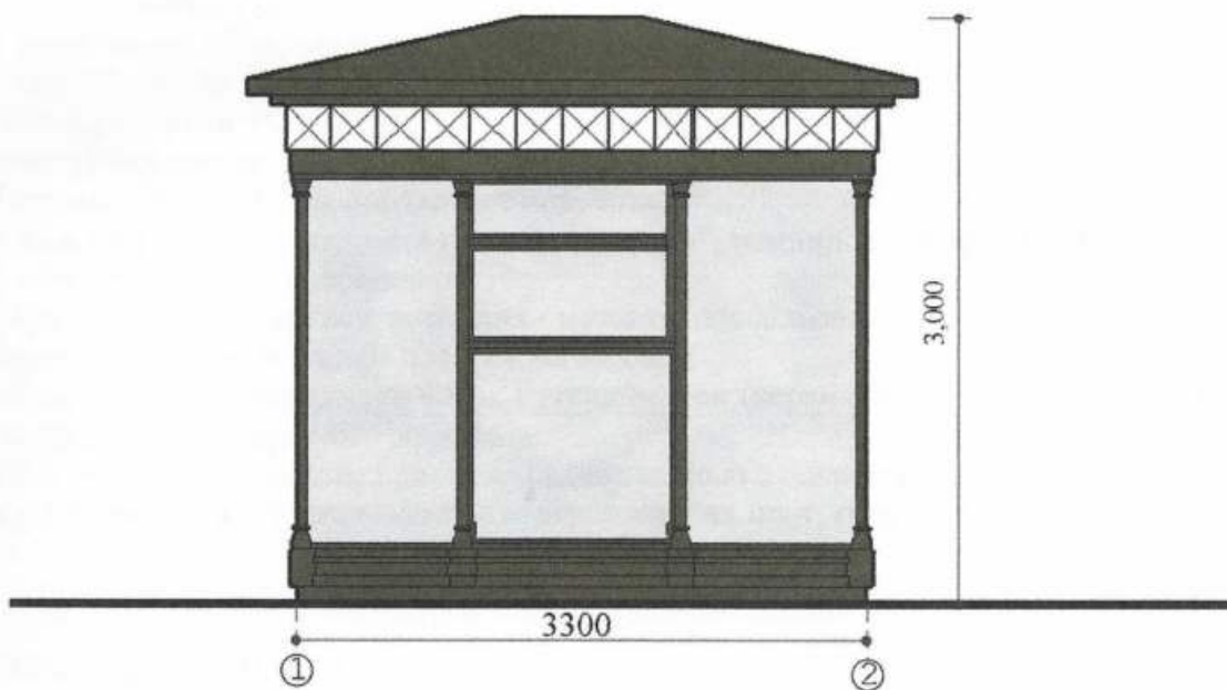
Боковий фасад
