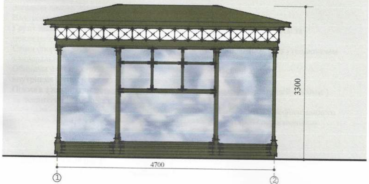
Боковий фасад
