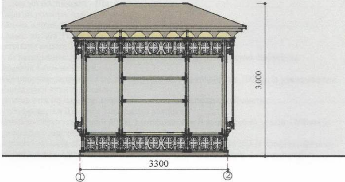
Головний фасад
