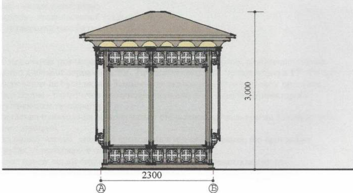
Боковий фасад
