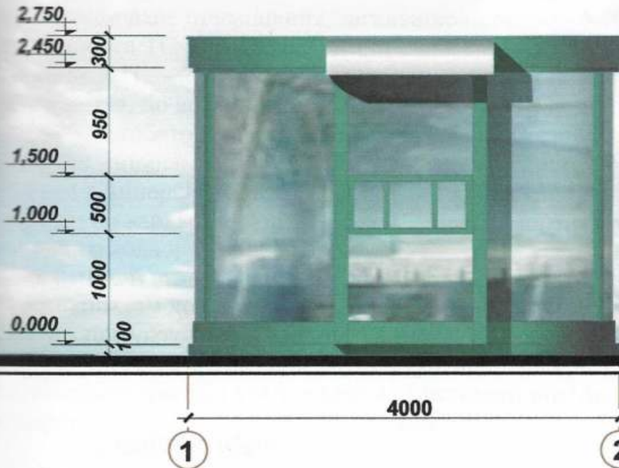
Бічний фасад
