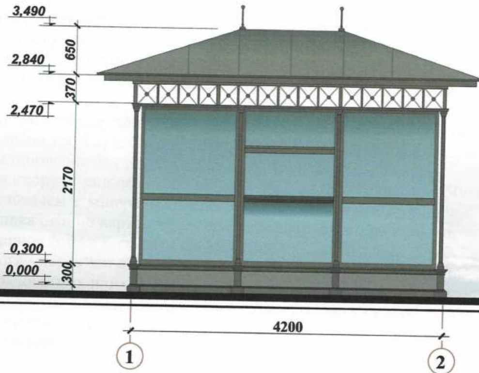
Головний фасад
