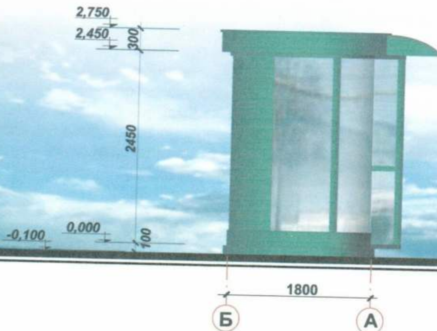
Боковий фасад
