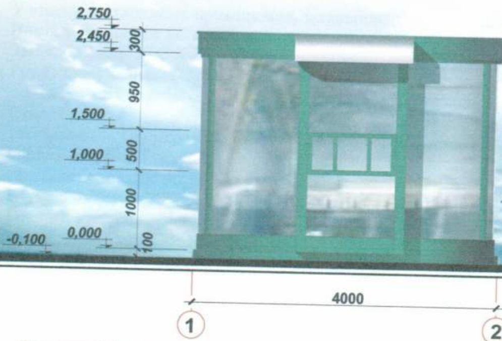
Боковий фасад
