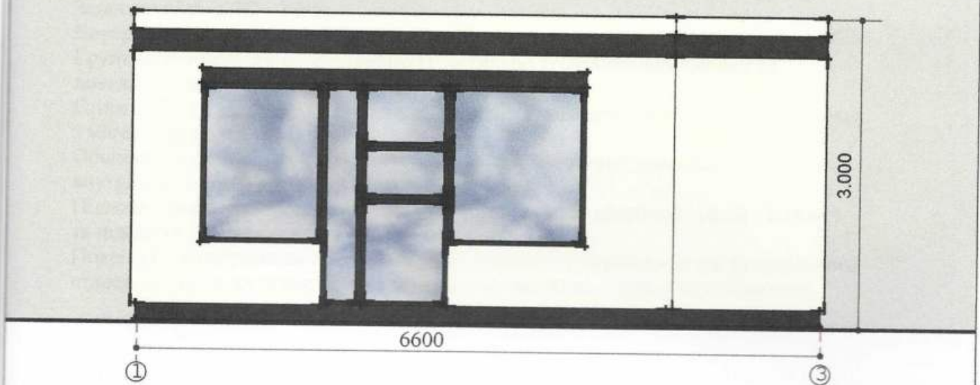
Боковий фасад
