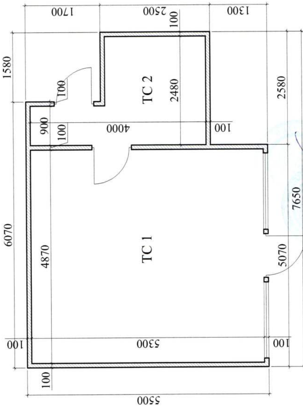
План ТСМ 1:50
