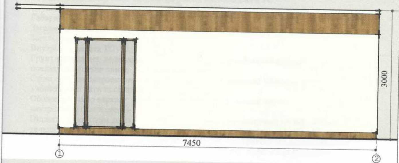
Боковий фасад
