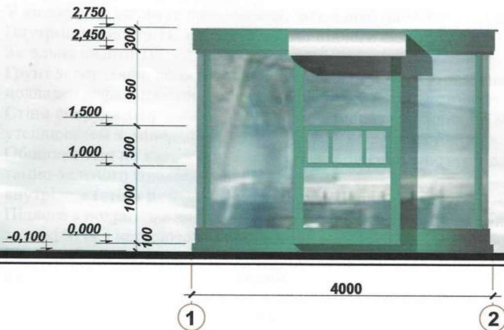
Бічний фасад
