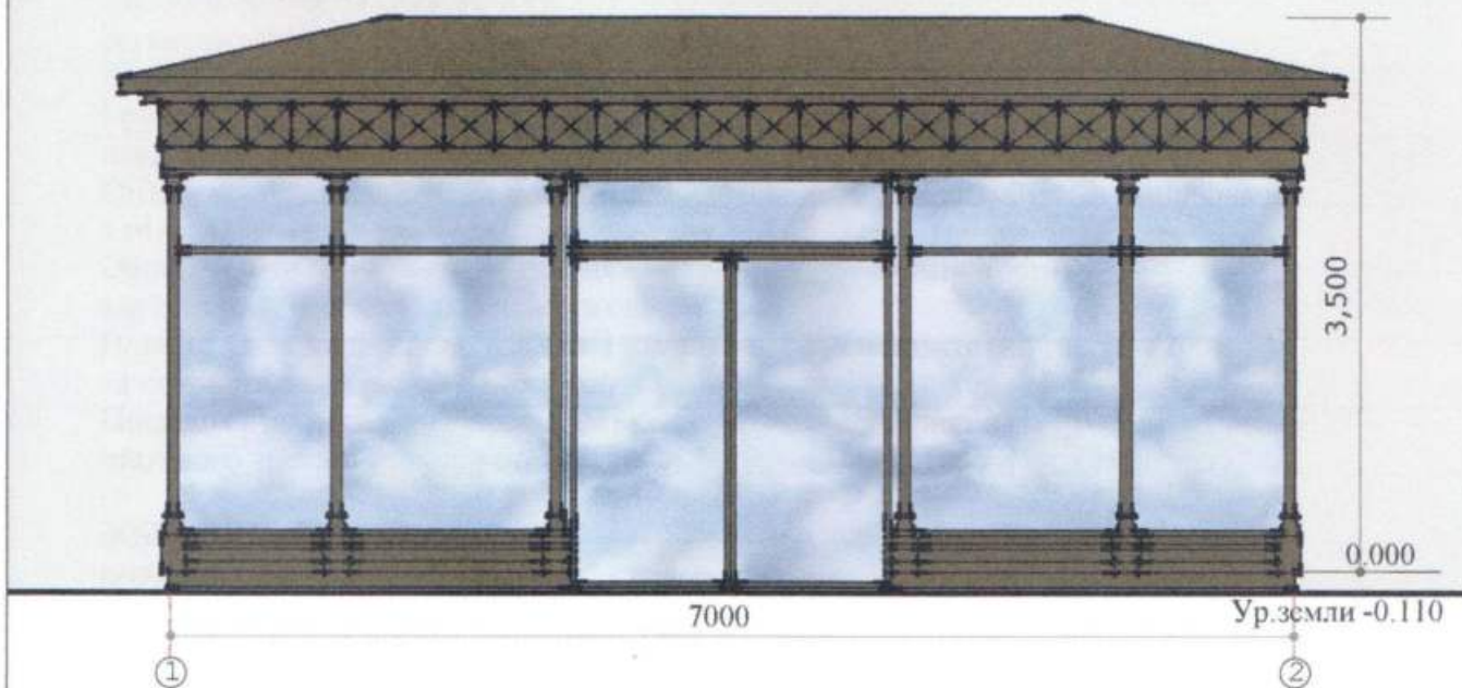
Боковий фасад
