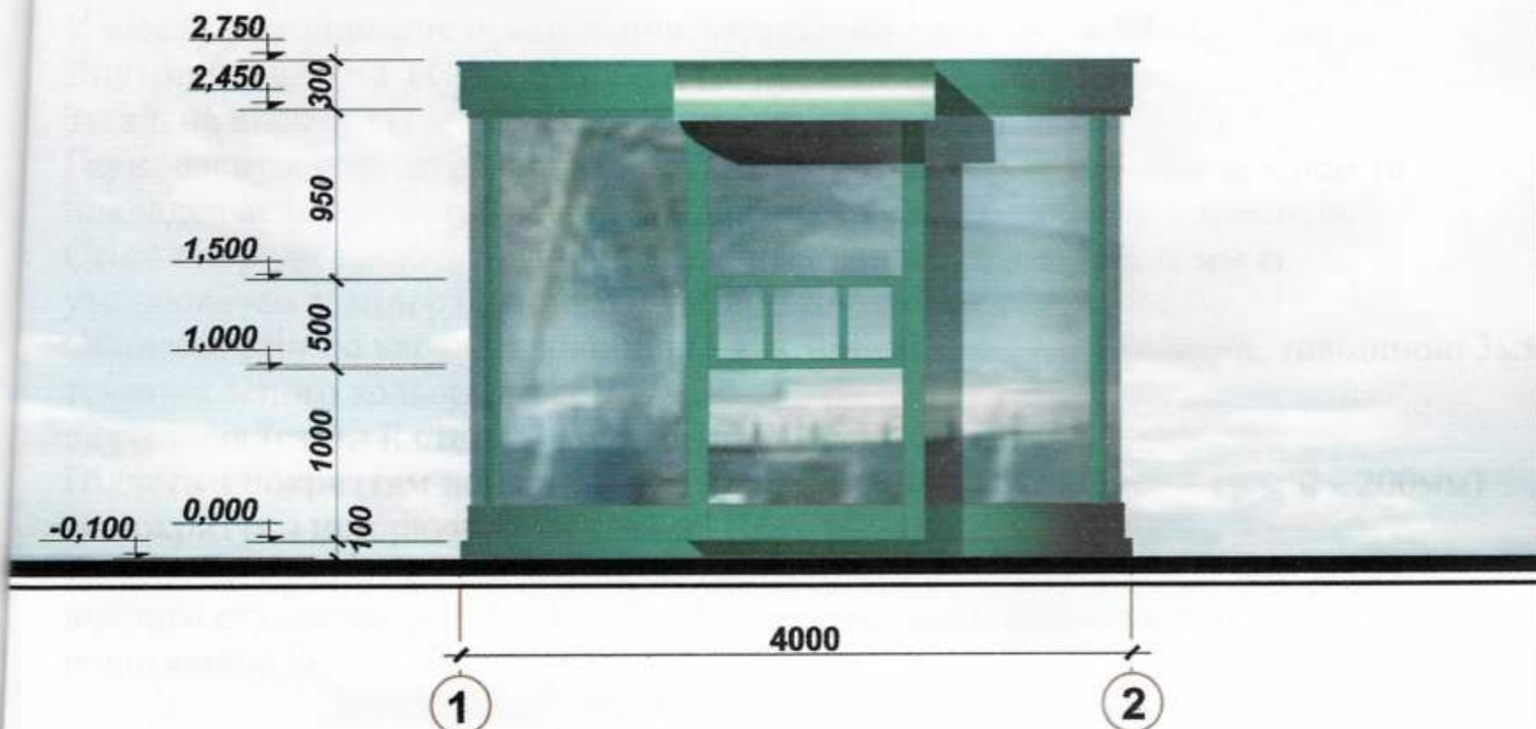
Бічний фасад
