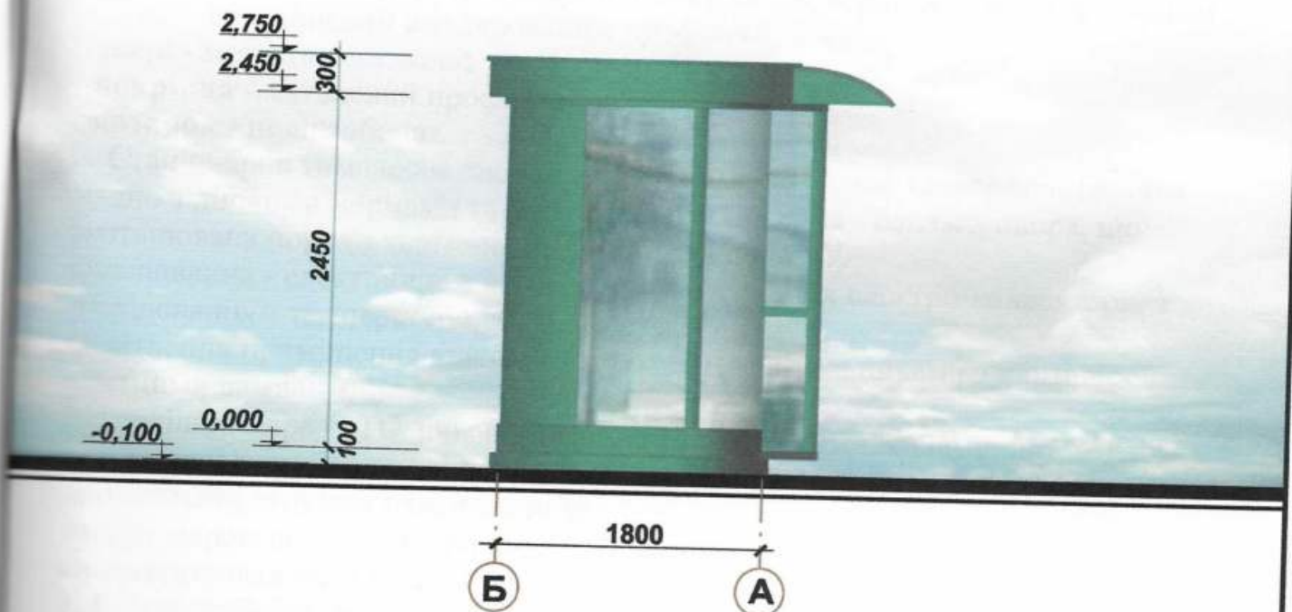
Бічний фасад
