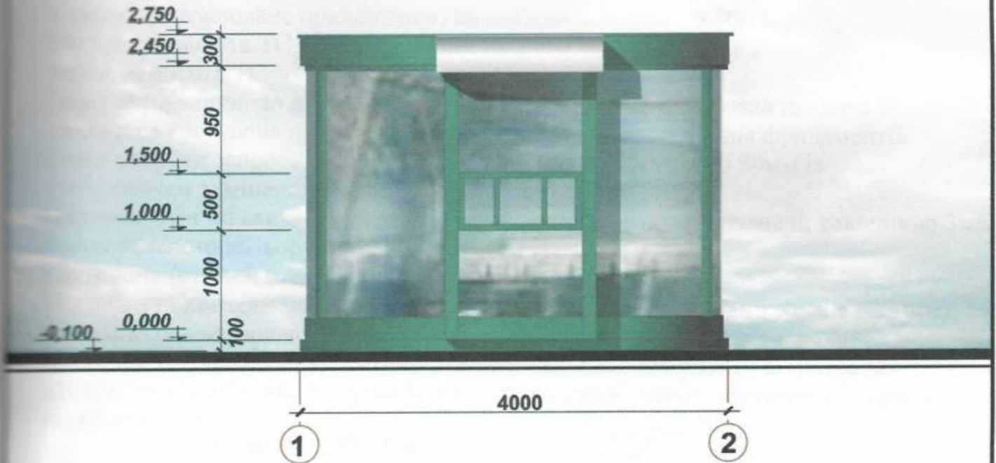
Бічний фасад
