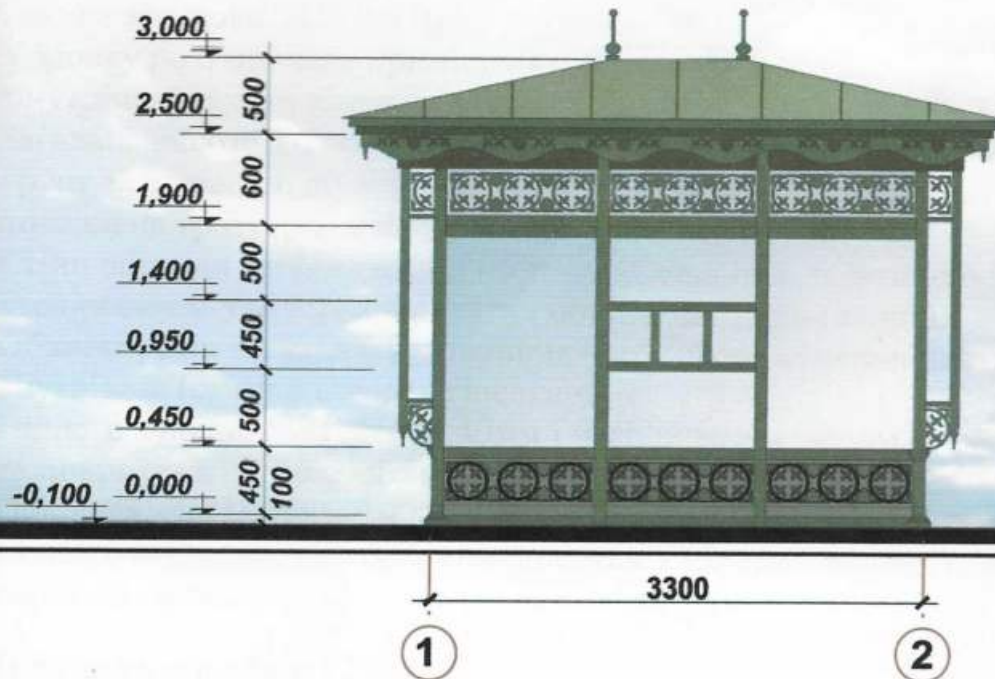
Бічний фасад
