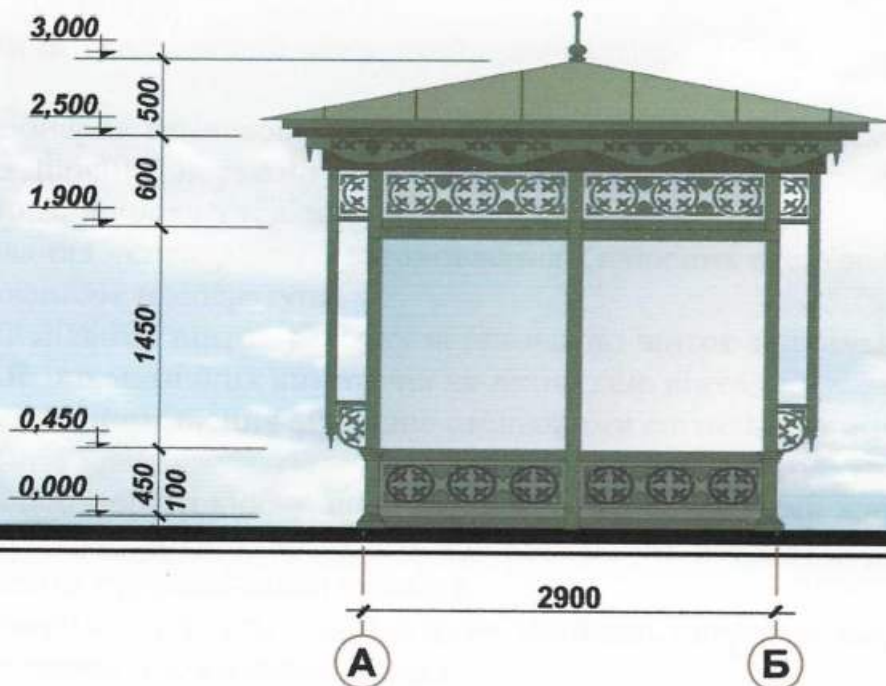
Бічний фасад
