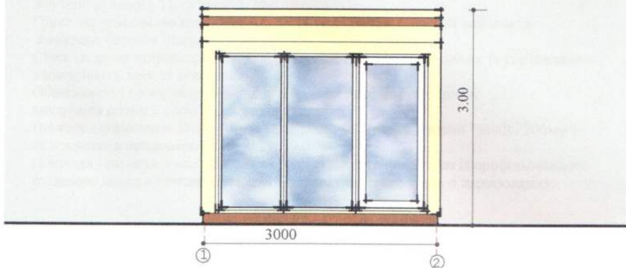
Боковий фасад
