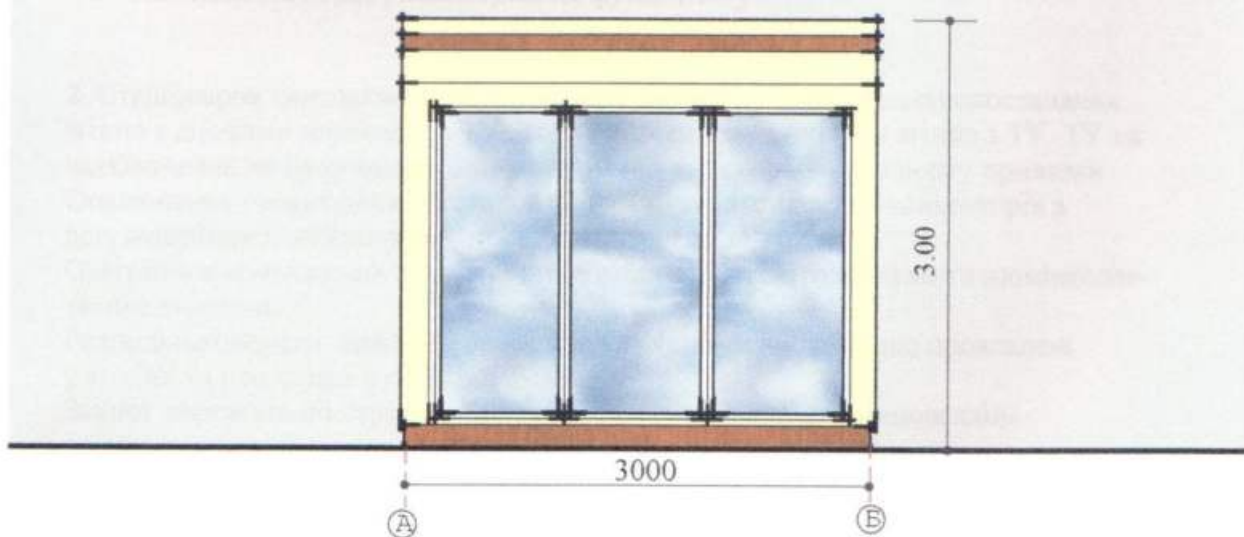
Боковий фасад
