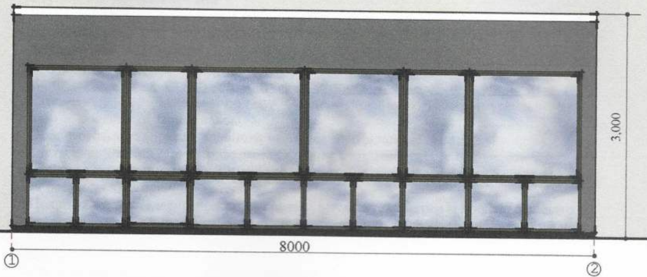
Боковий фасад
