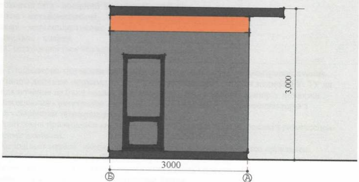
Боковий фасад
