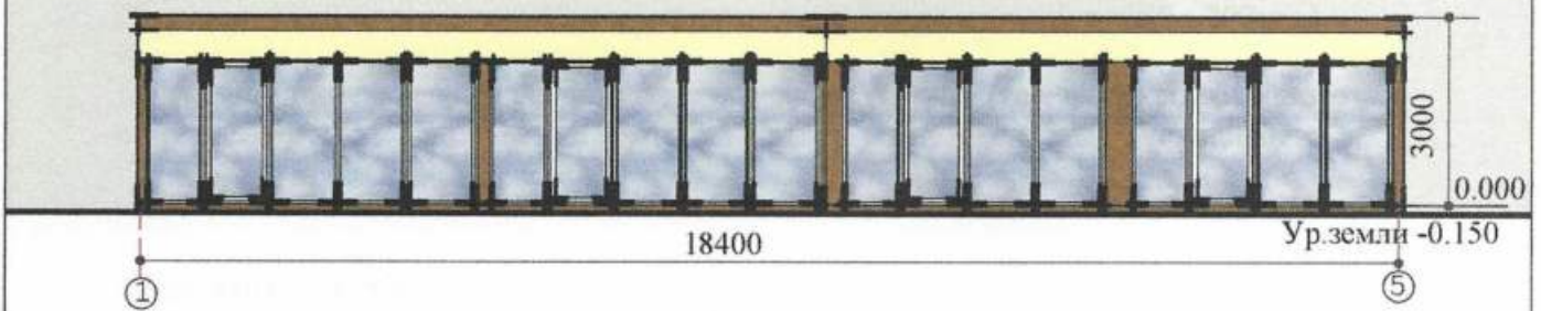
Боковий фасад
