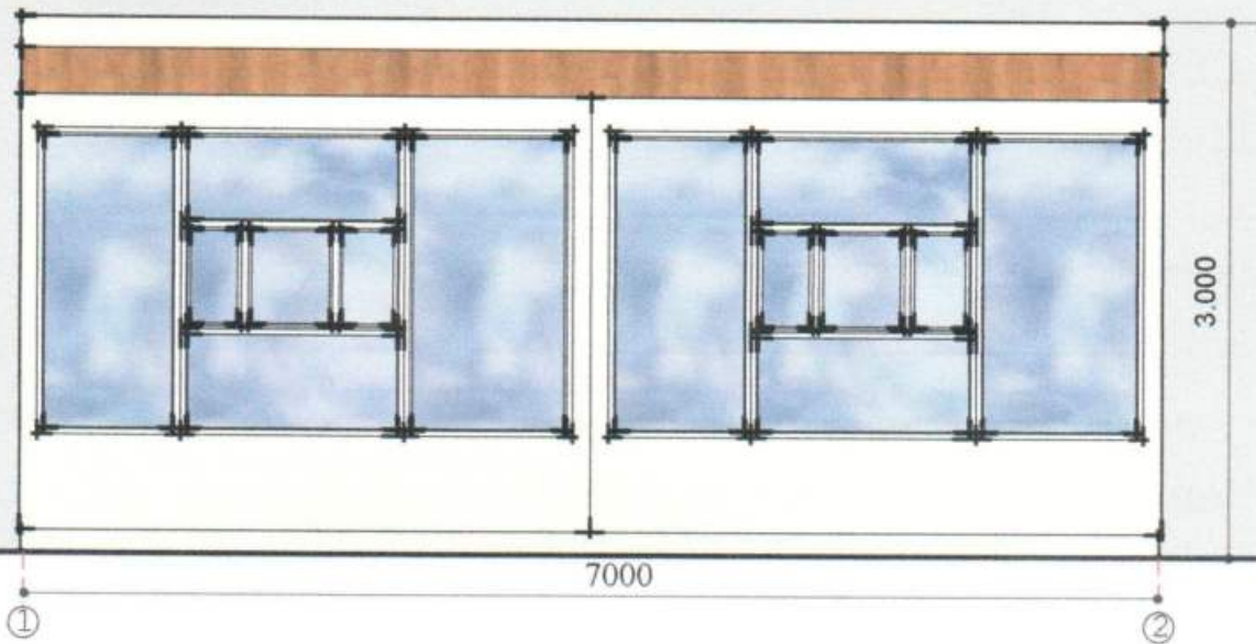
Боковий фасад
