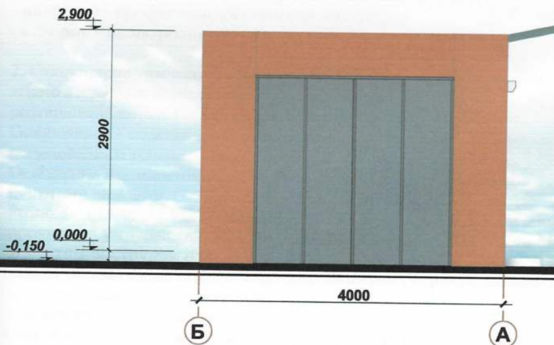
Бічний фасад
