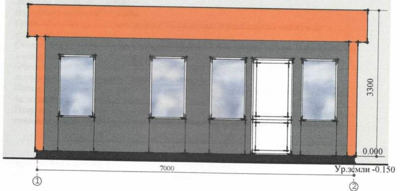
Боковий фасад
