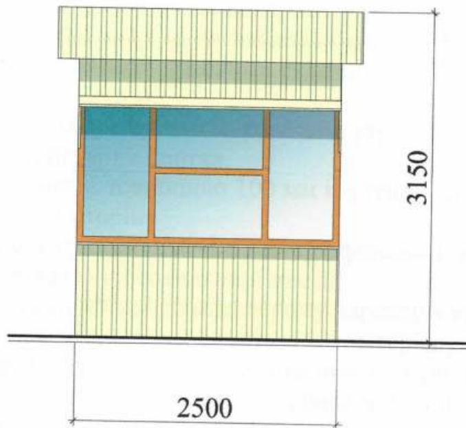
Бічний фасад М 1:50
