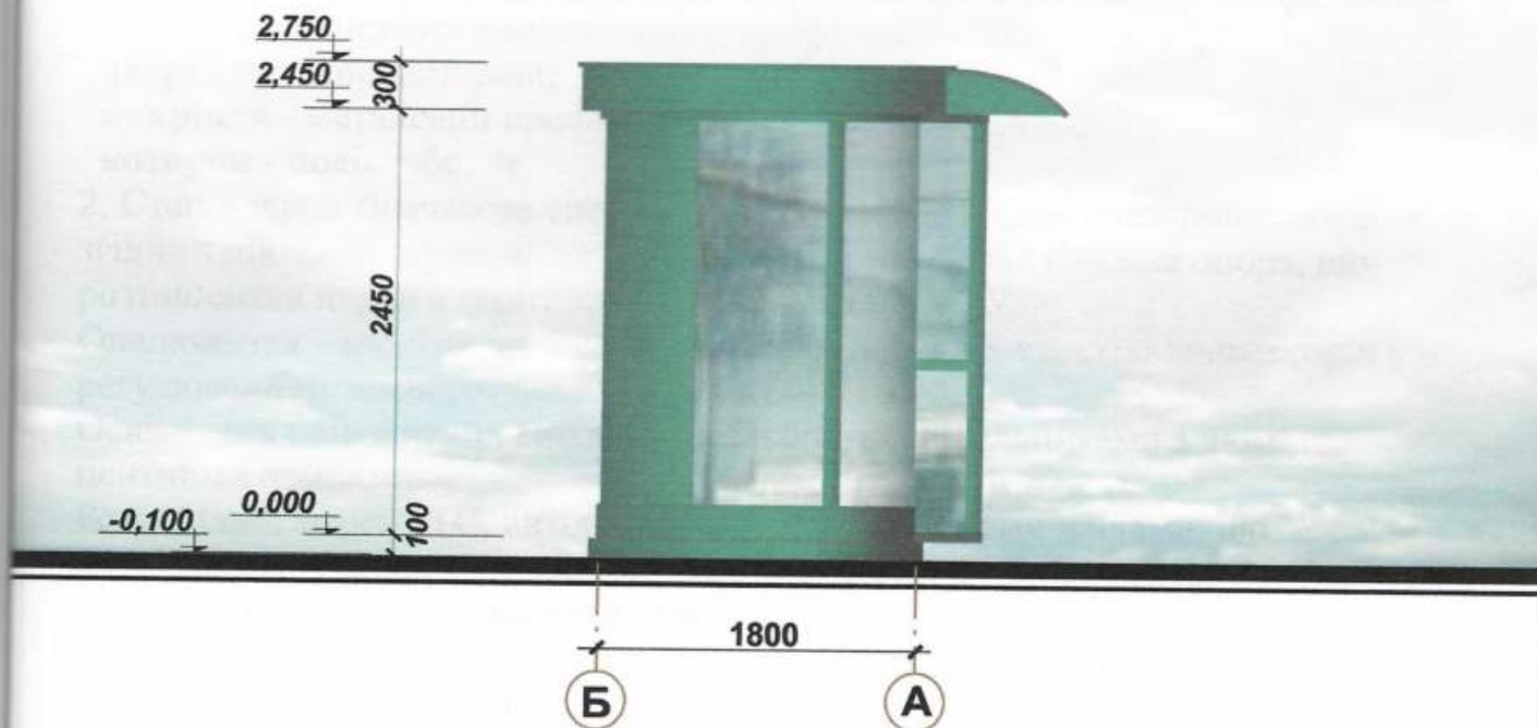
Бічний фасад
