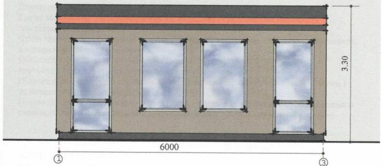
Боковий фасад
