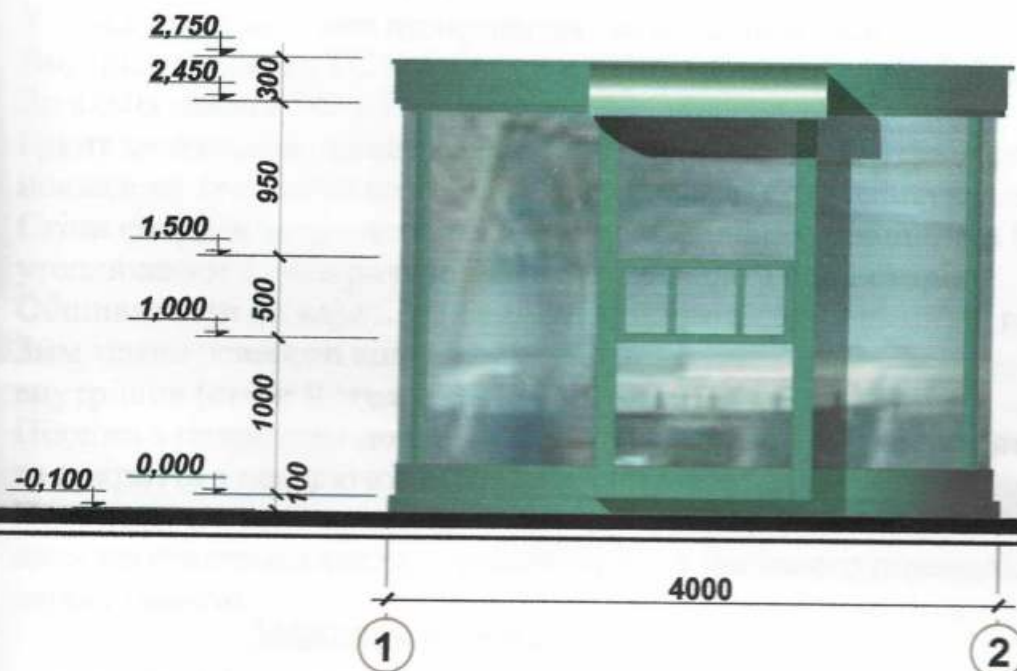
Бічний фасад
