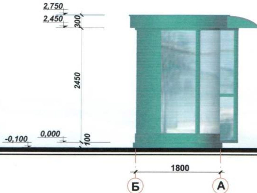
Бічний фасад
