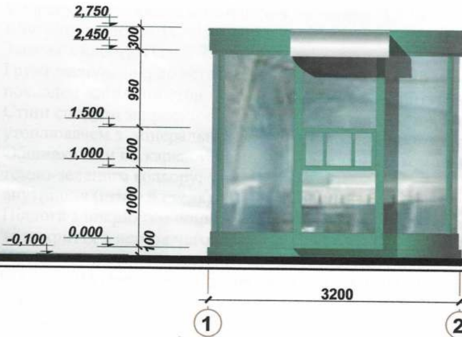
Бічний фасад
