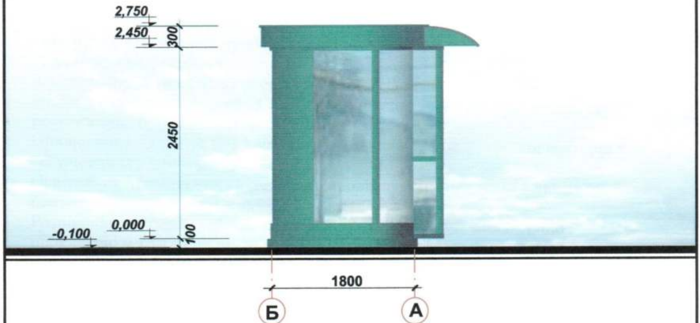
Бічний фасад
