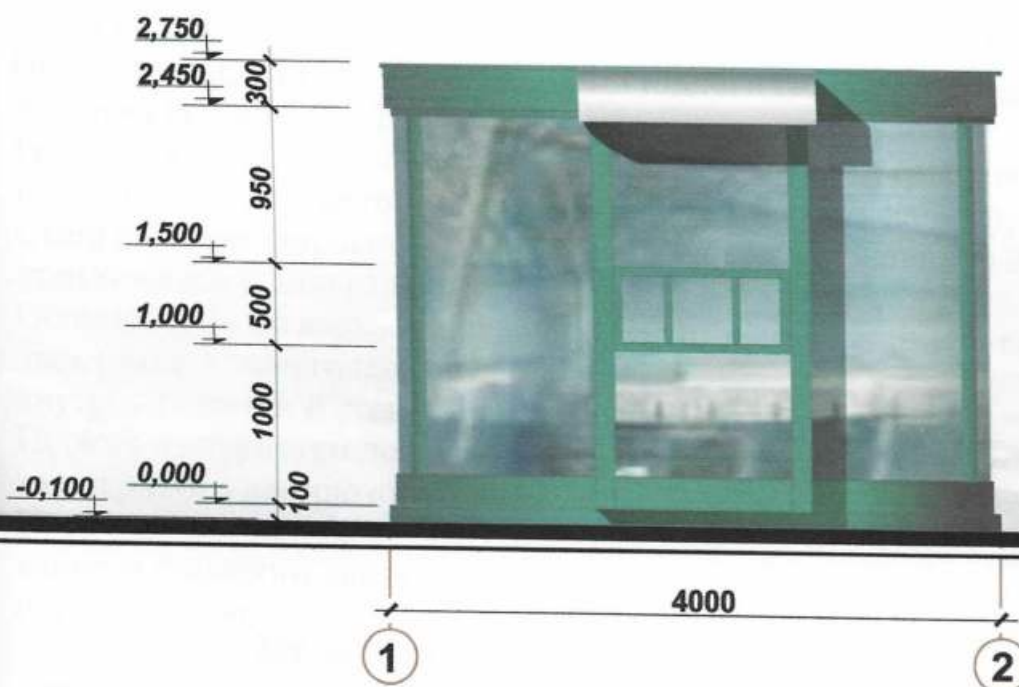
Бічний фасад
