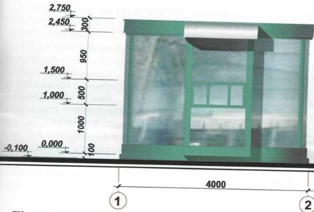
Бічний фасад
