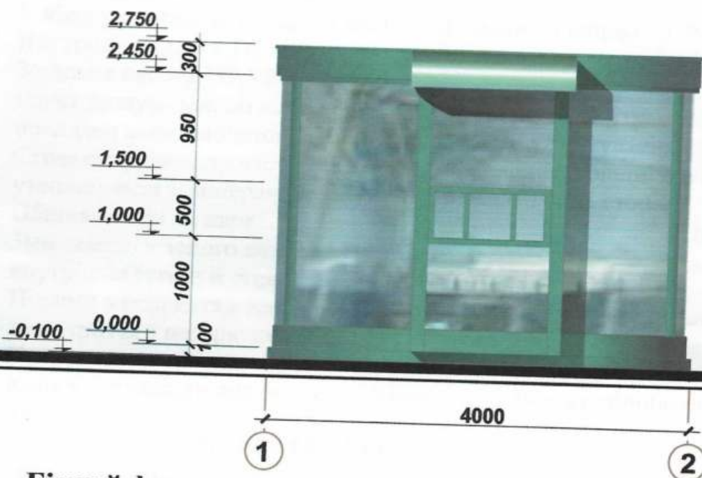
Бічний фасад
