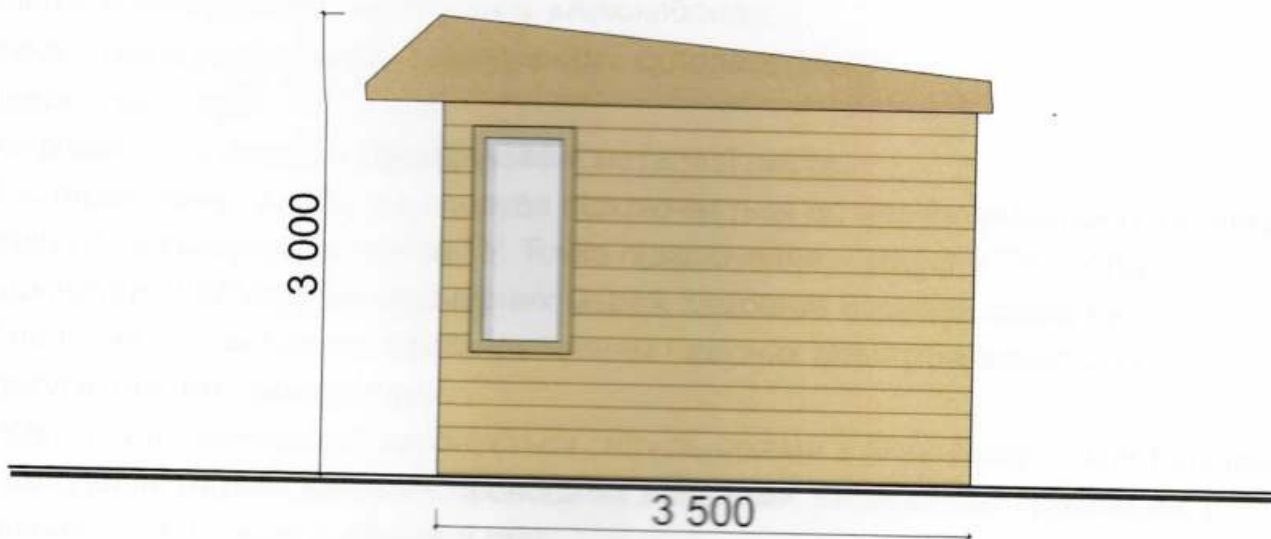
Бічний фасад
