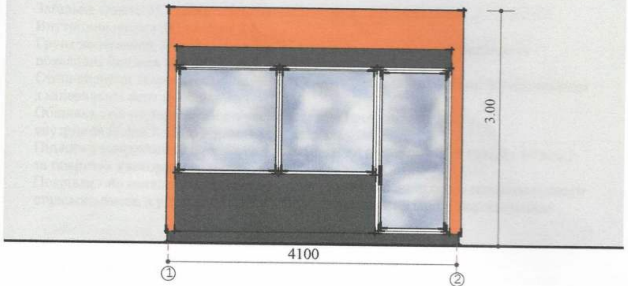
Боковий фасад
