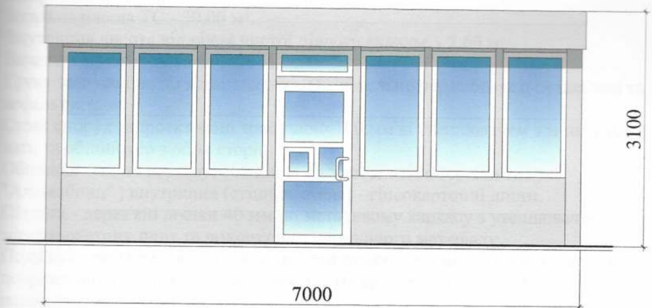
Бічний фасад ТС М 1:50
