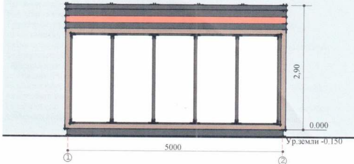
Боковий фасад
