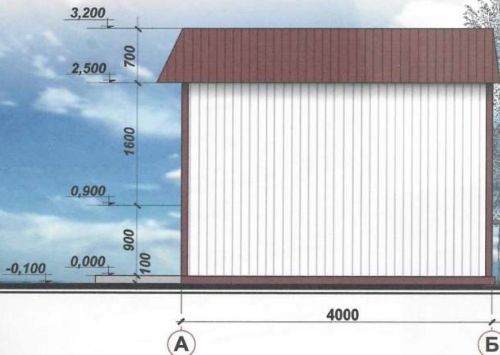
Боковий фасад М 1:50
