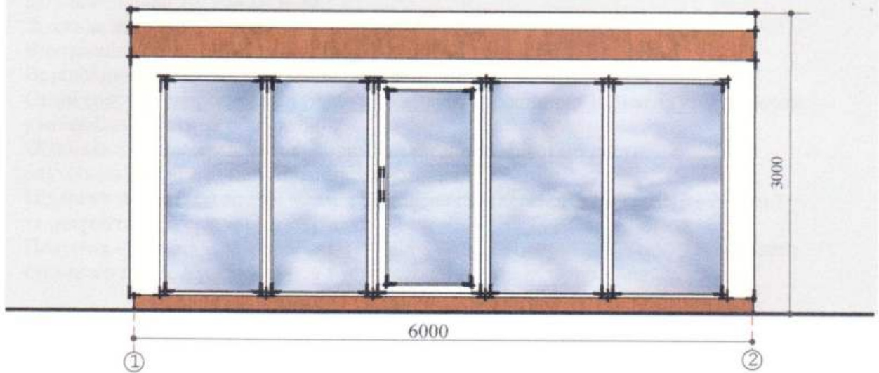
Боковий фасад
