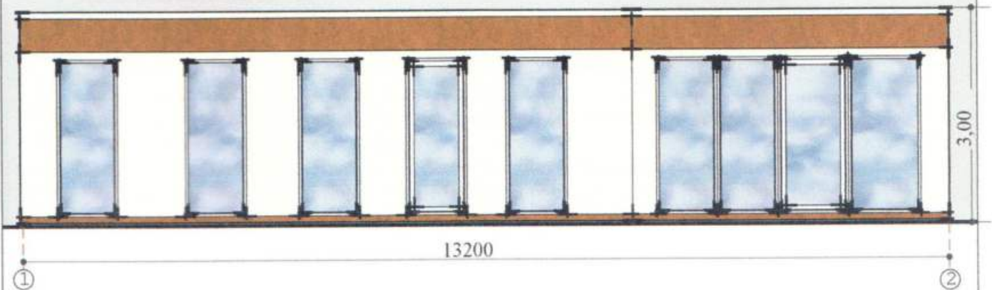
Боковий фасад м. 1:50
