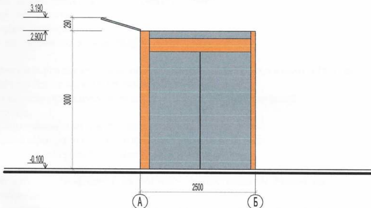
Фасад в осях "А"-"Б" М 1:50
