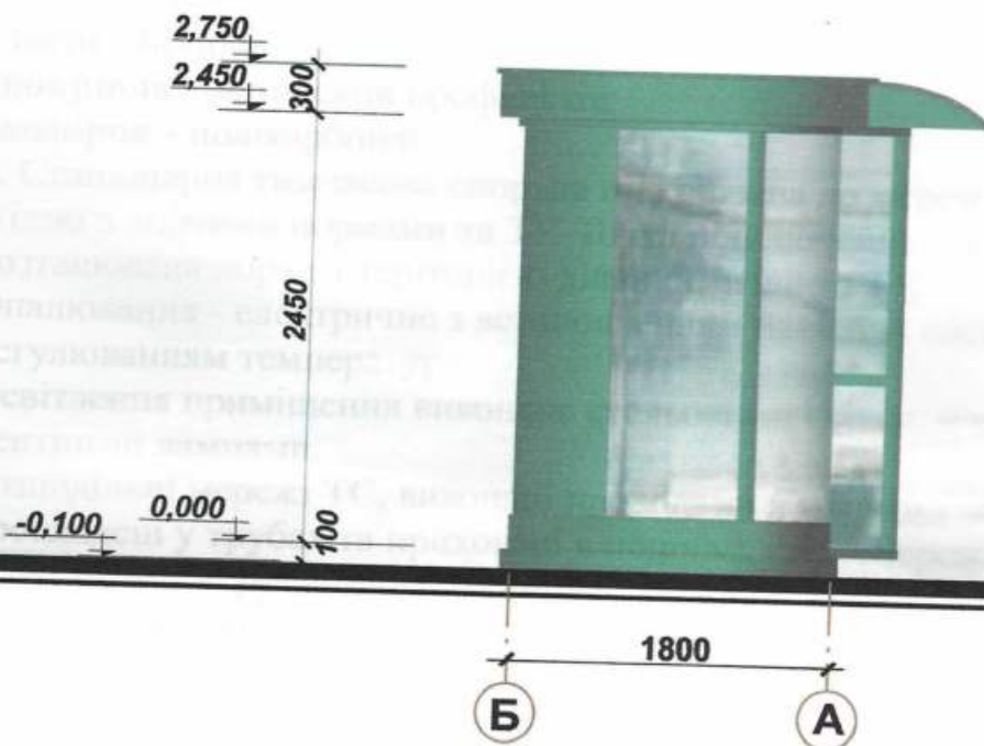
Бічний фасад
