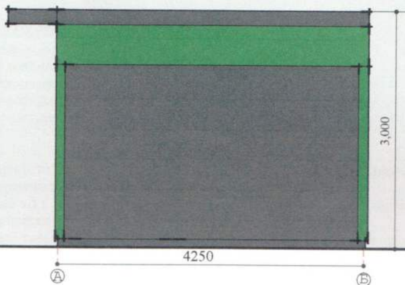
Боковий фасад
