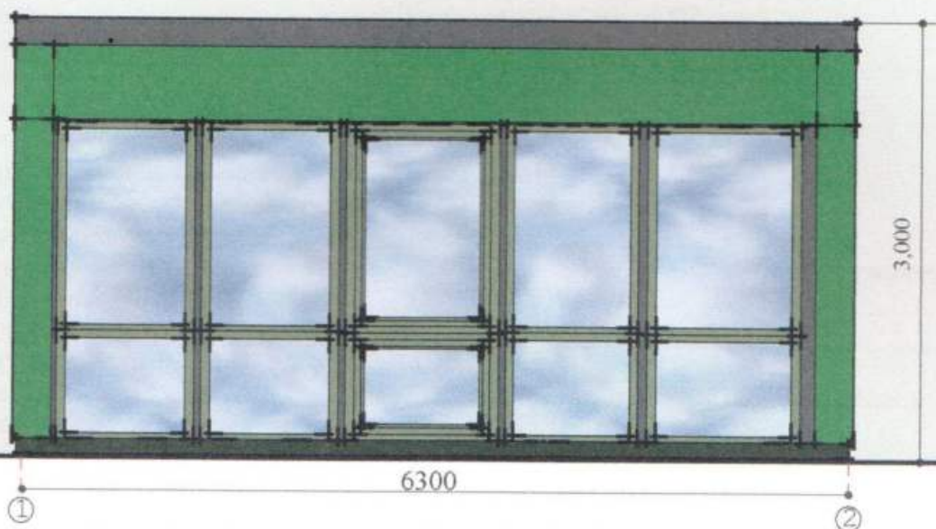
Головний фасад
