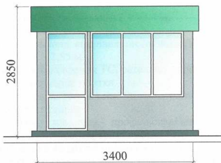
Головний фасад М 1:50
