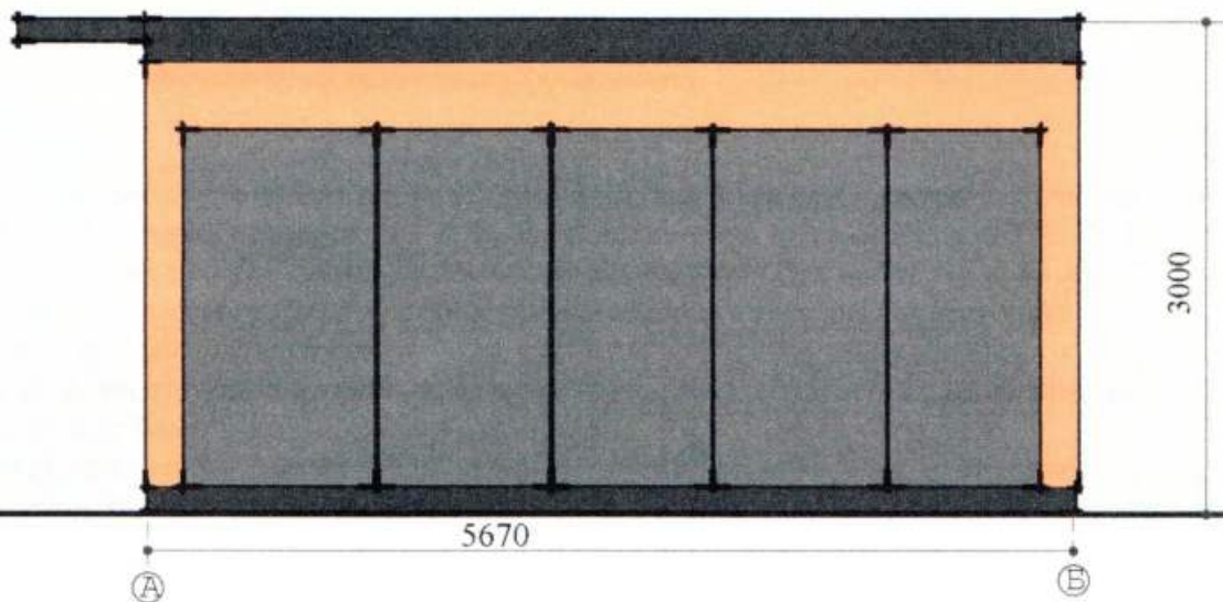
Боковий фасад
